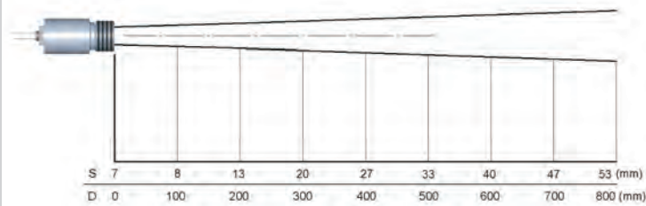
15:1 optics
