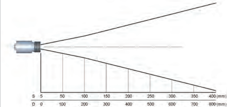
2:1 optics
