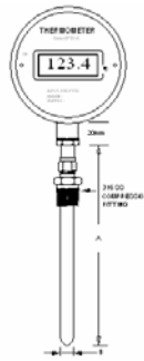
DWG: SD 385
